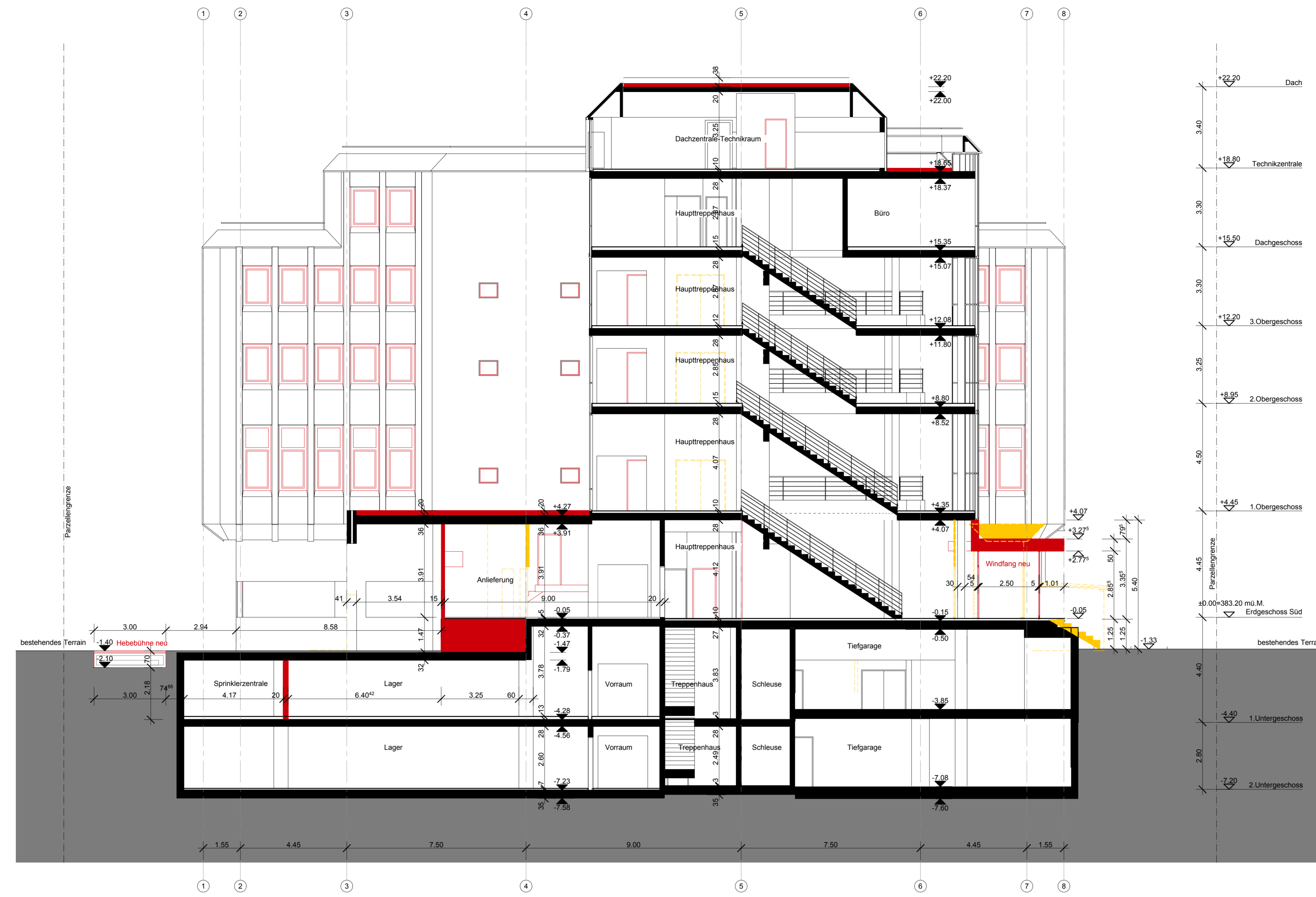
Schnitt C-C
