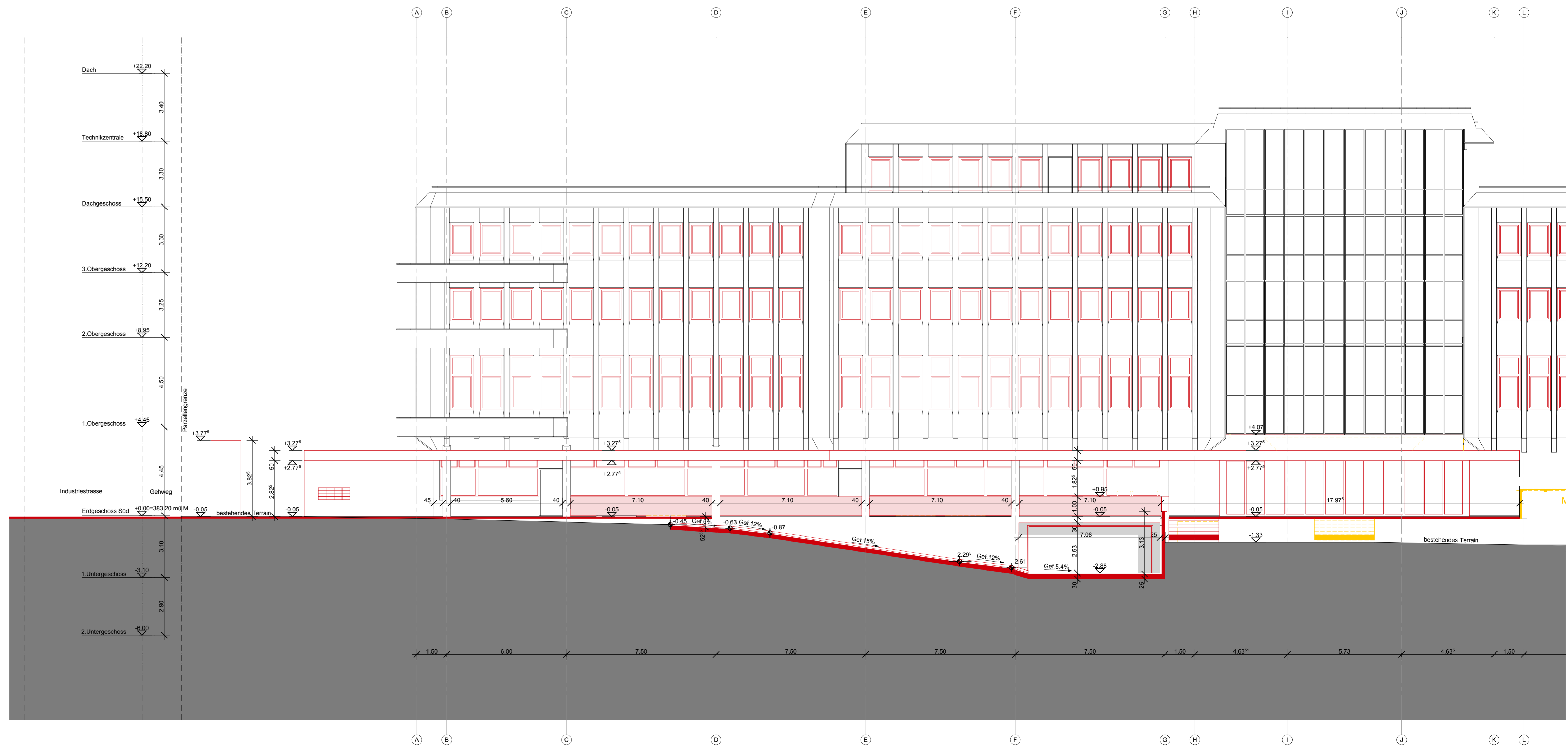
Schnitt E-E
