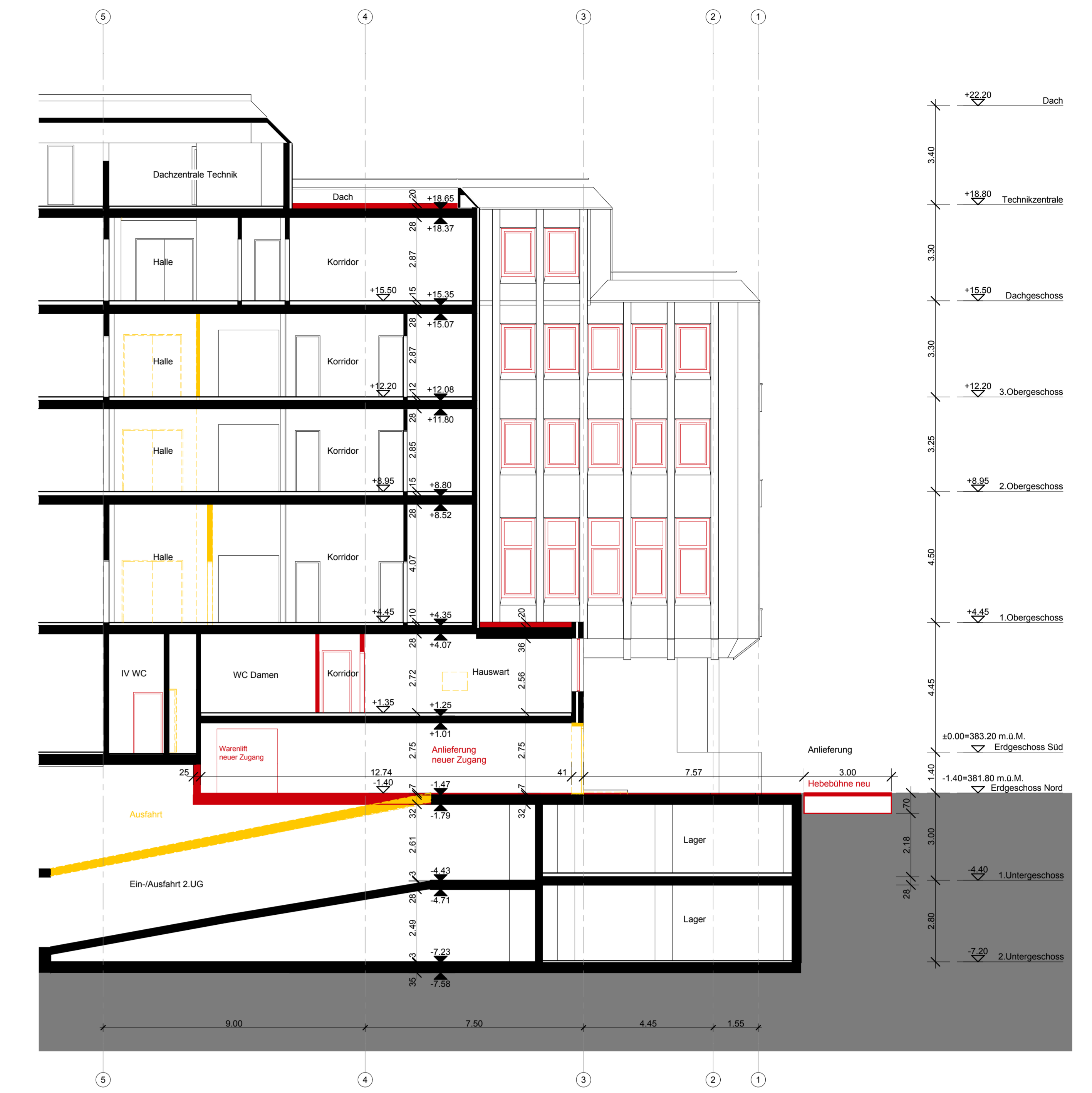
Schnitt D-D
