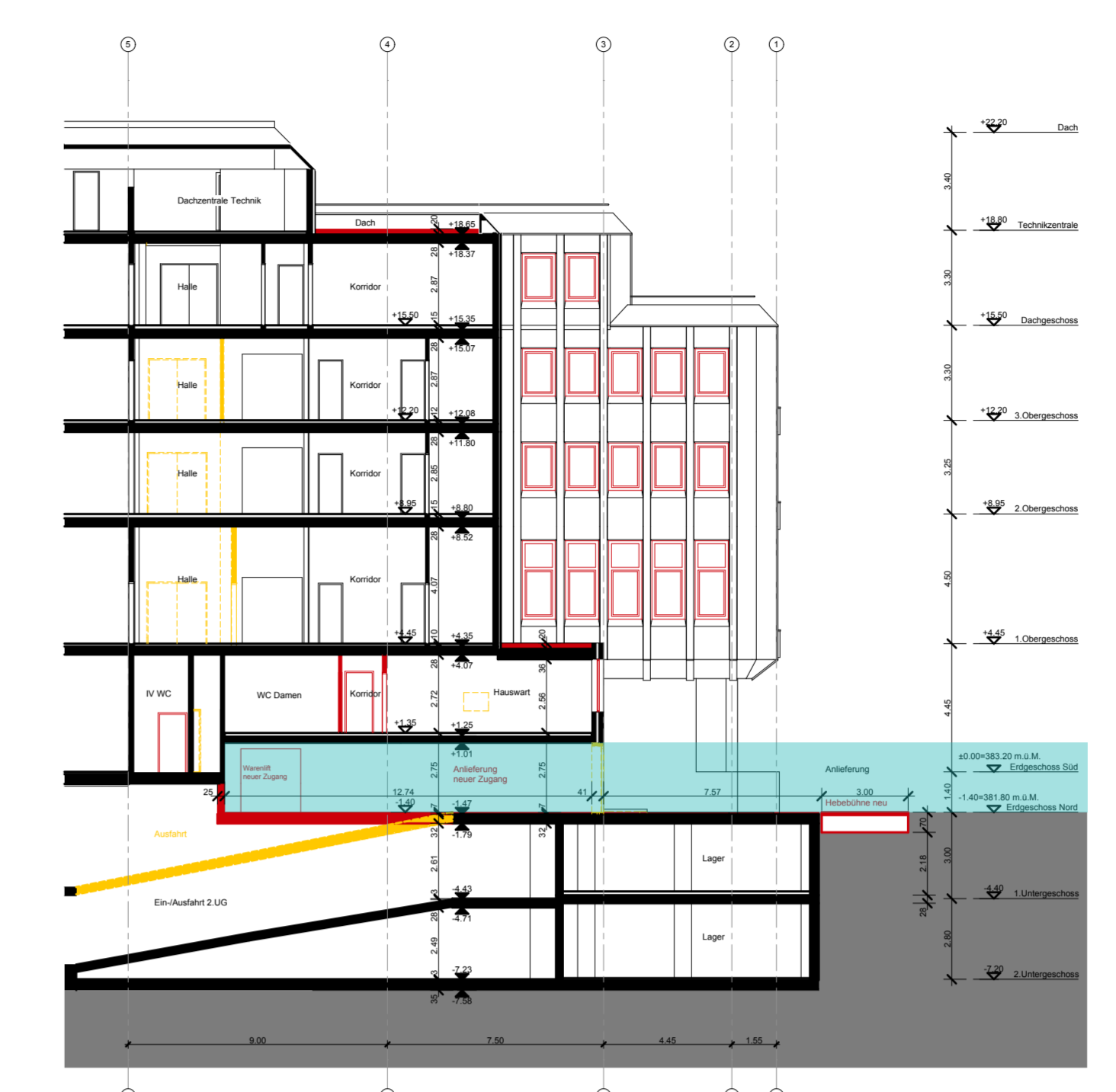
Schnitt D-D 1:200
